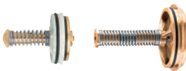
Instroomkeerklep voor series 574 en 575. Clapet amont pour séries 574 et 575.
