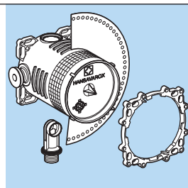
muurinbouwkast voor het kraanlichaam, art. nr. 616.030.00.1
